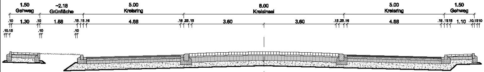
Querschnitt
